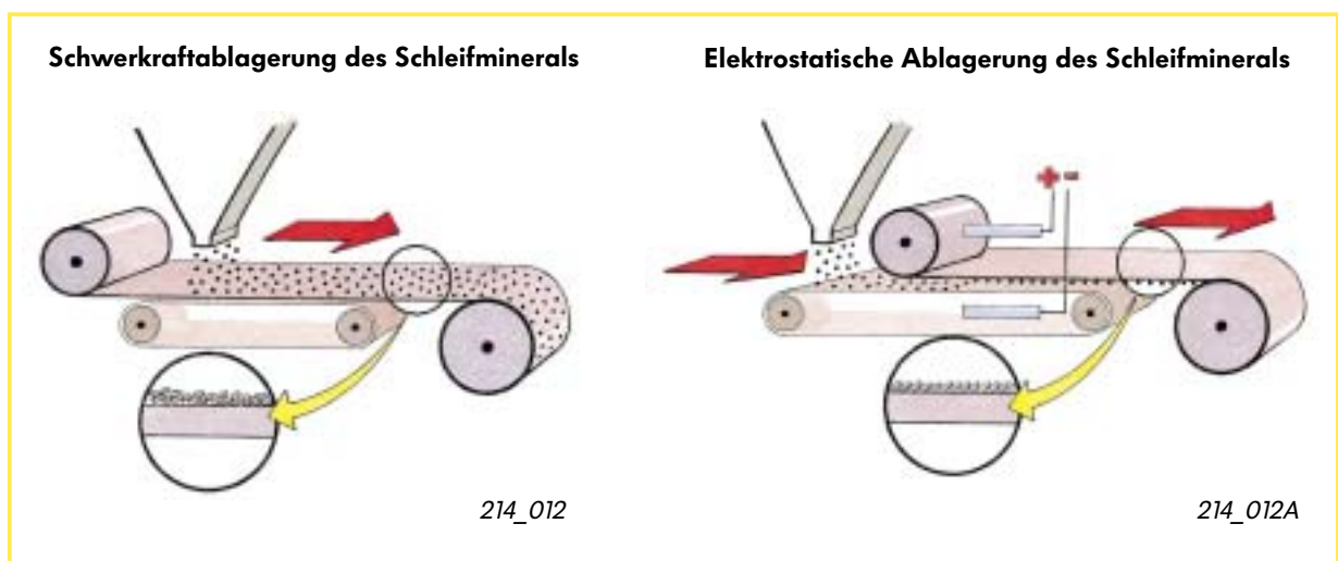
Schwerkraftauftrag und elektrostatischer Auftrag
