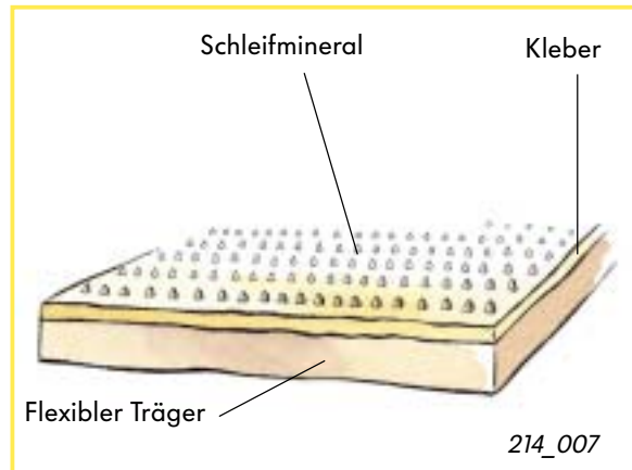
Aufbau der Schleifmittel
